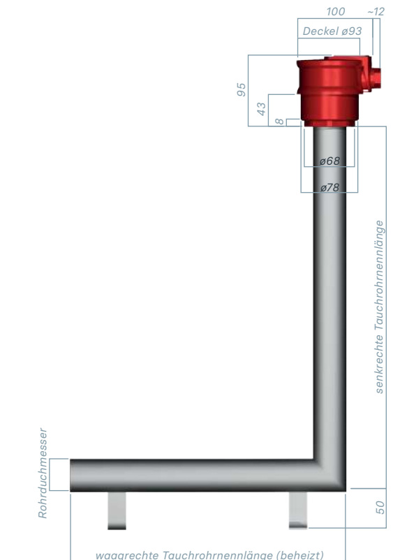
Winkelbadwärmer ROTKAPPE
